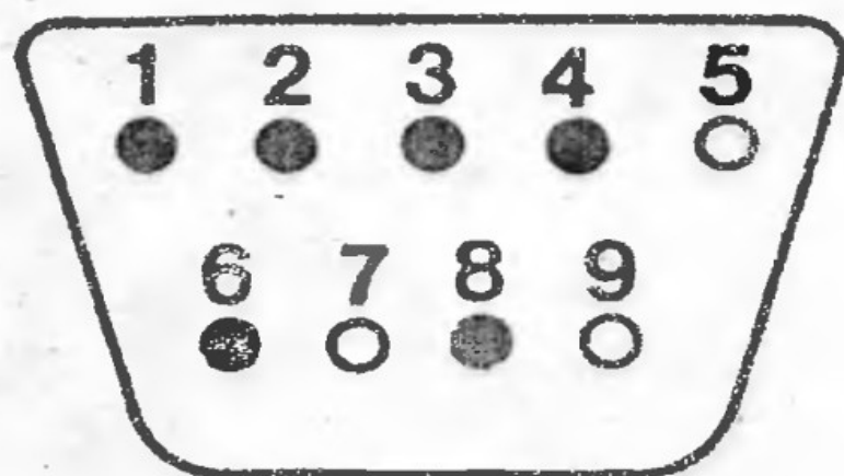
Rys. 5. Standardowy wtyk połączeniowy
