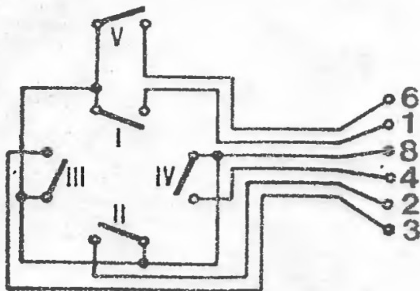
Rys. 6. Schemat elektryczny układu drążka
