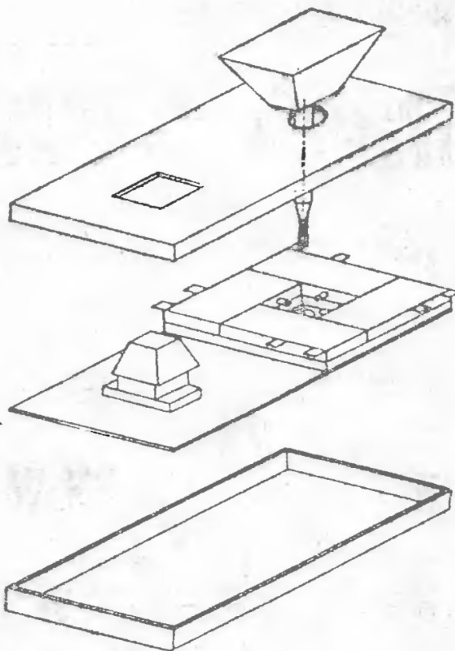
Rys. 4. Drążek sterowy, sposób montażu
