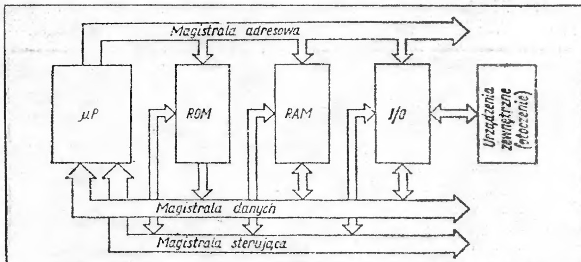
Schemat blokowy komputera
