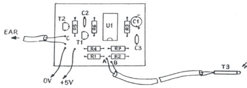
Rys. 4 — Rozmieszczenie elementów na płytce.
