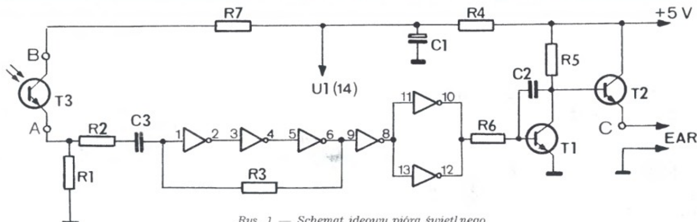
Rys. 1 — Schemat ideowy pióra świetlnego.
