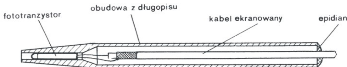
Rys. 2 — Konstrukcja mechaniczna pióra.
