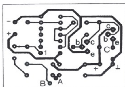
Rys. 3 — Płytka drukowana wzmacniacza sygnału.
