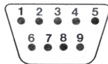
Rys. 4. Wtyczka Eltra 881, widok od strony połączeń lutowicznych.
