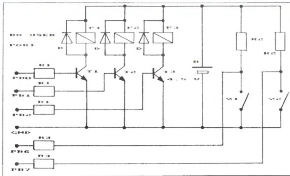
Rys. 1 Schemat układu sterującego samochodzikiem.
