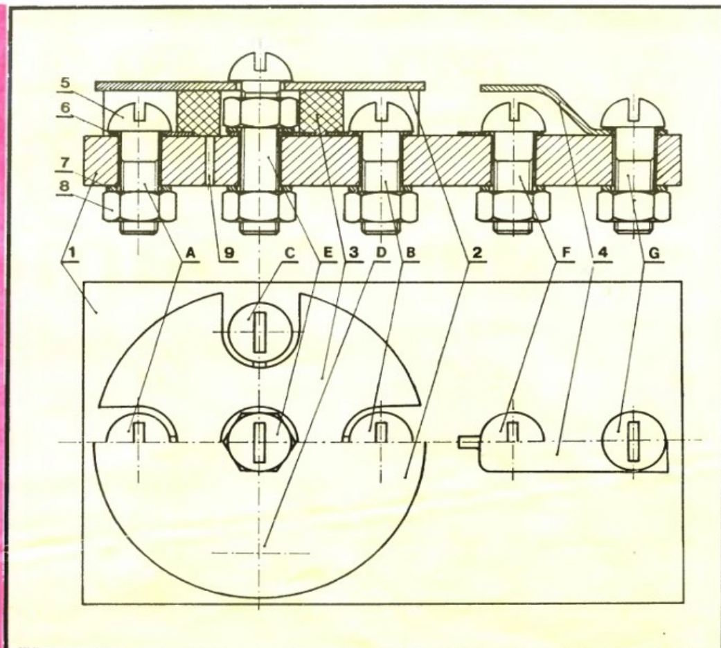
Rys. 1. Konstrukcja manipulatora: 1 — podstawa, 2 — blaszka, 3 — gąbka, 4 — styk sprężysty „fire”, 5 — wkręty z łbami okrągłymi (7 sztuk), 6 — podkładka stykowa (7 sztuk), 7 — podkładka zwykła (8 sztuk), nakrętka ośmiokątna (8 sztuk), 9 — otwór na przewody elektryczne.
