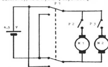
Rys. 2 Połączenie przekaźników z silniczkami.
