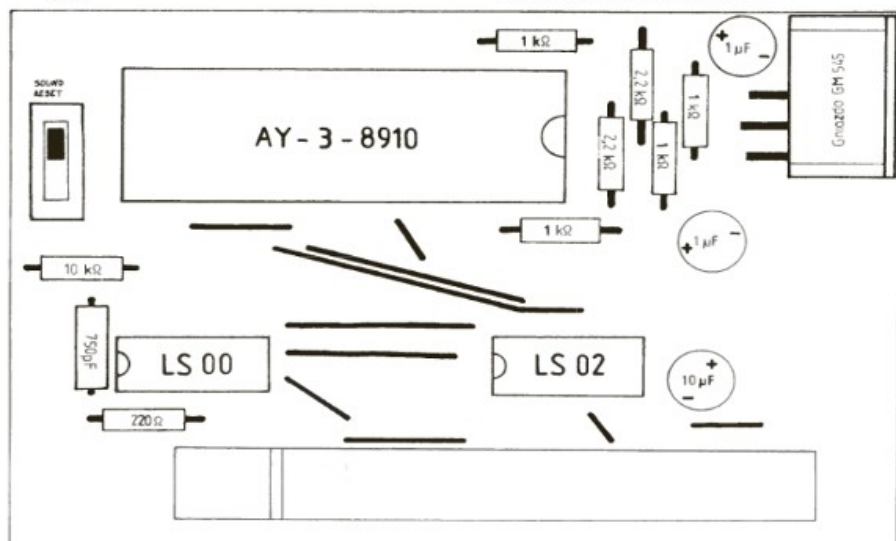
Rys.1 Widok elementów AY-3-8910 SOUND INTERFACE
