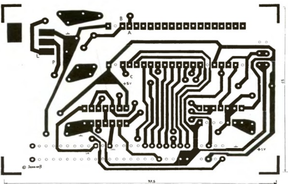
Rys. 2 Widok płytki do AY-3-8910 SOUND INTERFACE
