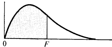
The F -distribution
