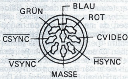
So ist die DIN-Buchse mit dem Monitorausgang beim MZ700 beschaltet
