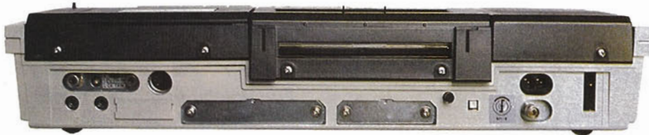
Die Rückseite des MZ700 besitzt Ausgänge für TV, Monitor und den Systembus (abgedeckt)
