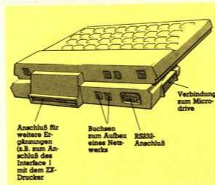
Bild 3. Schema des Interface 1 mit den Anschlüssen
