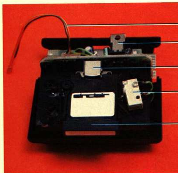
Bild 8a. Wenn der Schreibschutz aus der Kassettenseite herausgebrochen worden ist, sperrt ein Mikroswitcher (an der rechten Seite des Schachts) den Schreibteil.
