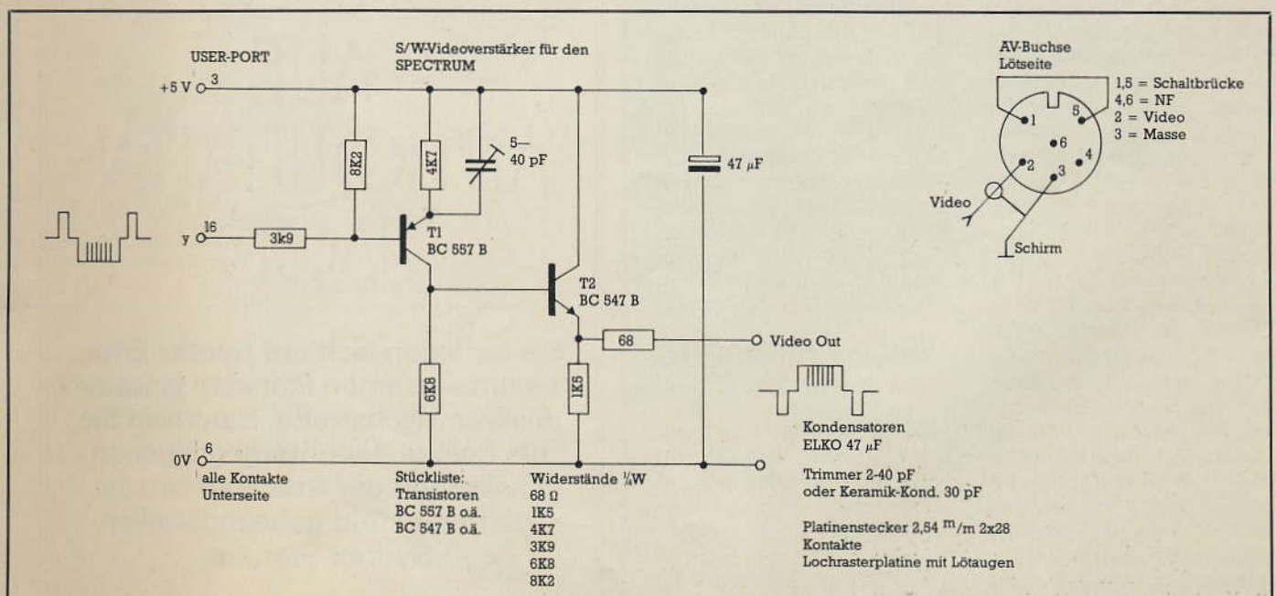
Schaltung Videoausgang
