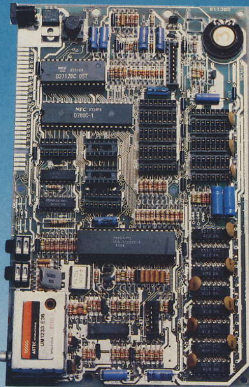
Bild 2. Die 16-KByte-Platine Typ 3
